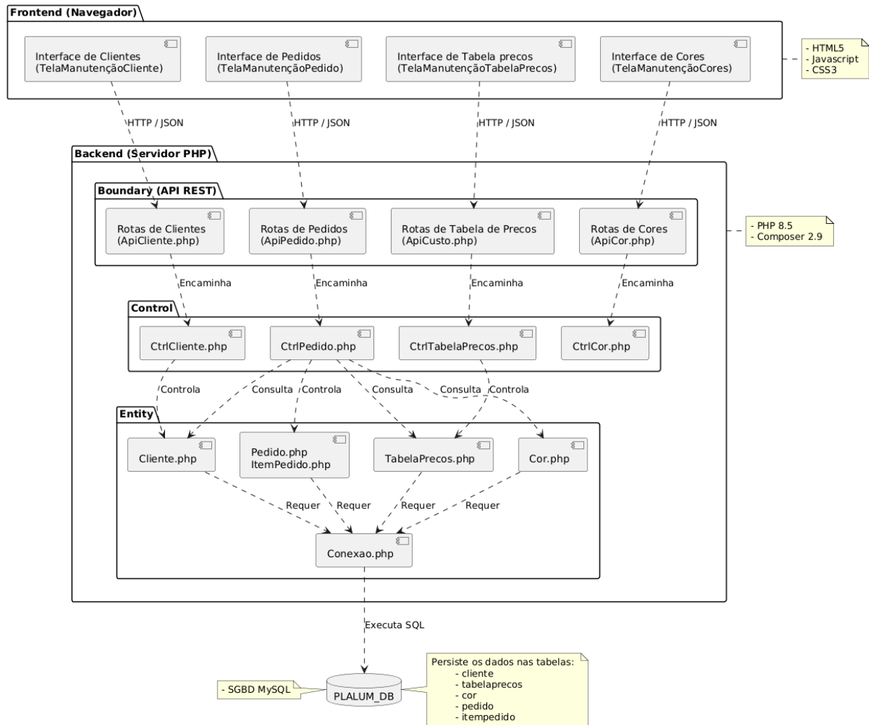
Diagrama de Componentes Atualizado
